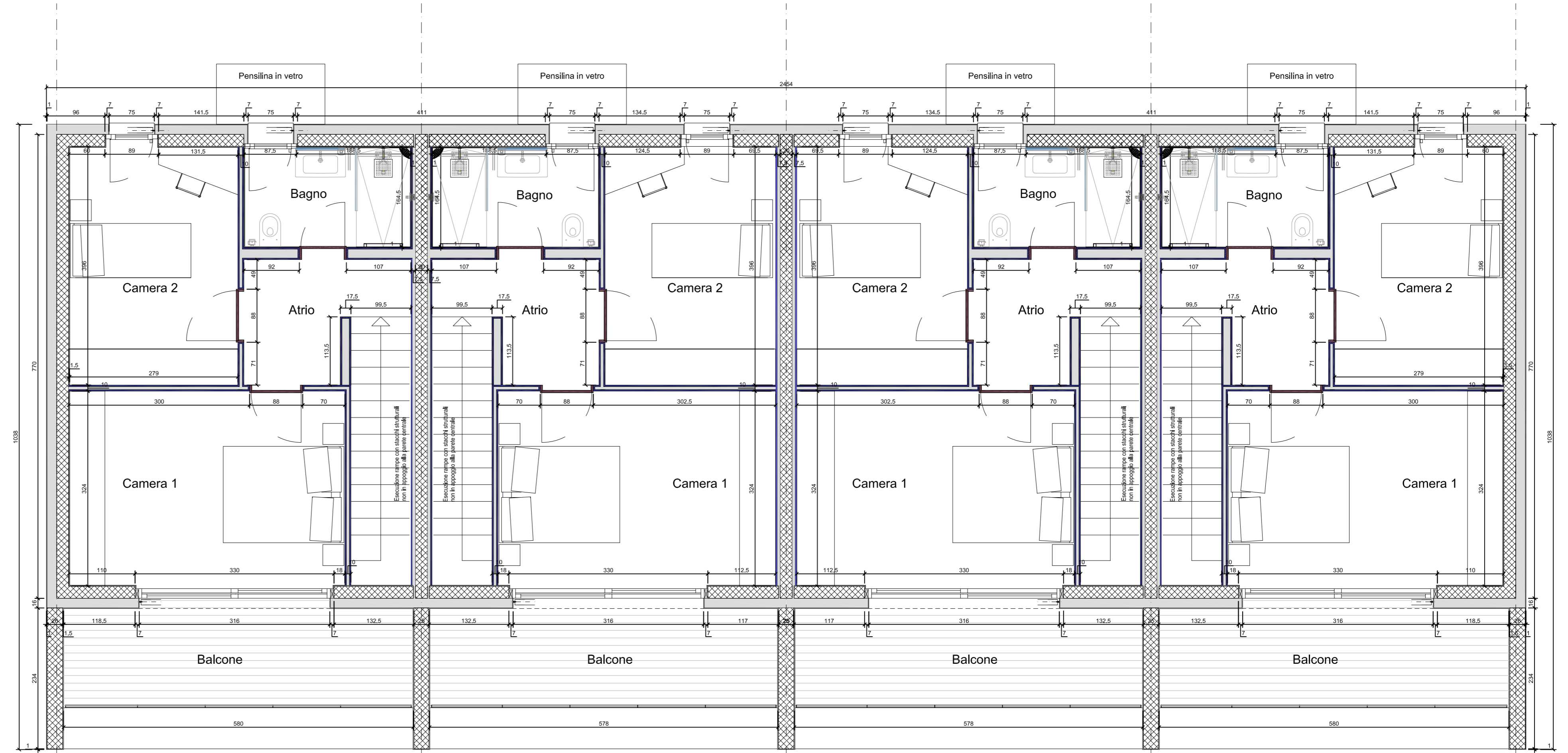
PIANO PRIMO
